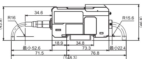
ZP-L30□および延長ケーブル(XS3W-M421/M423-□-R)接続時
