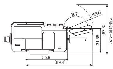
カバー、ボタン開位置(DINレール取付)
