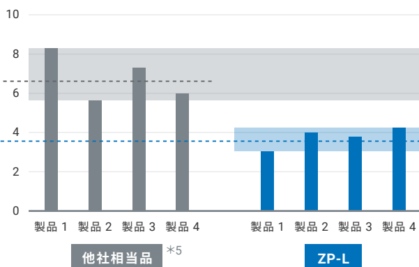
移動時の測定値のばらつき (移動分解能) [ \mu m]
