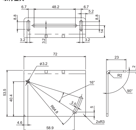
取付金具
